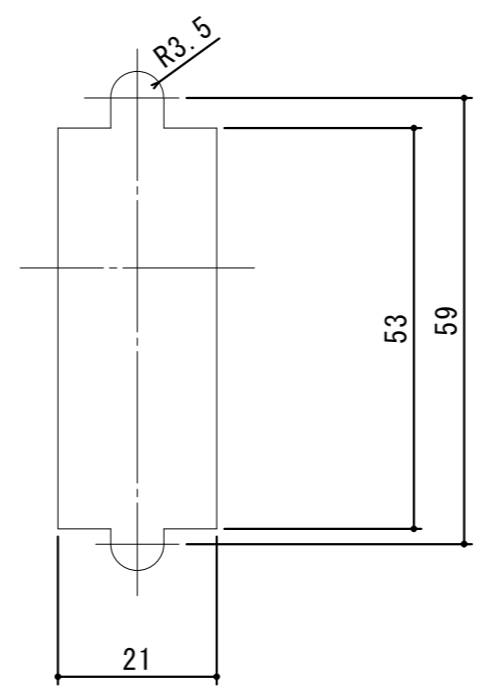
パネル穴明け寸法
