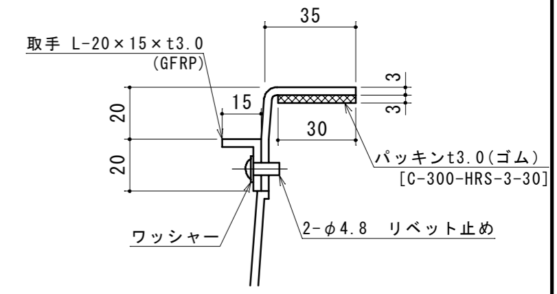
A 詳細図 S=1:2
