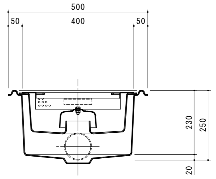
A 詳細図 S=1:2
