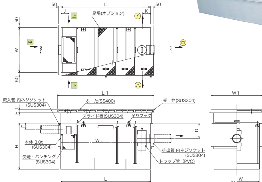
構造図
