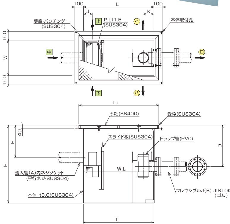
構造図
