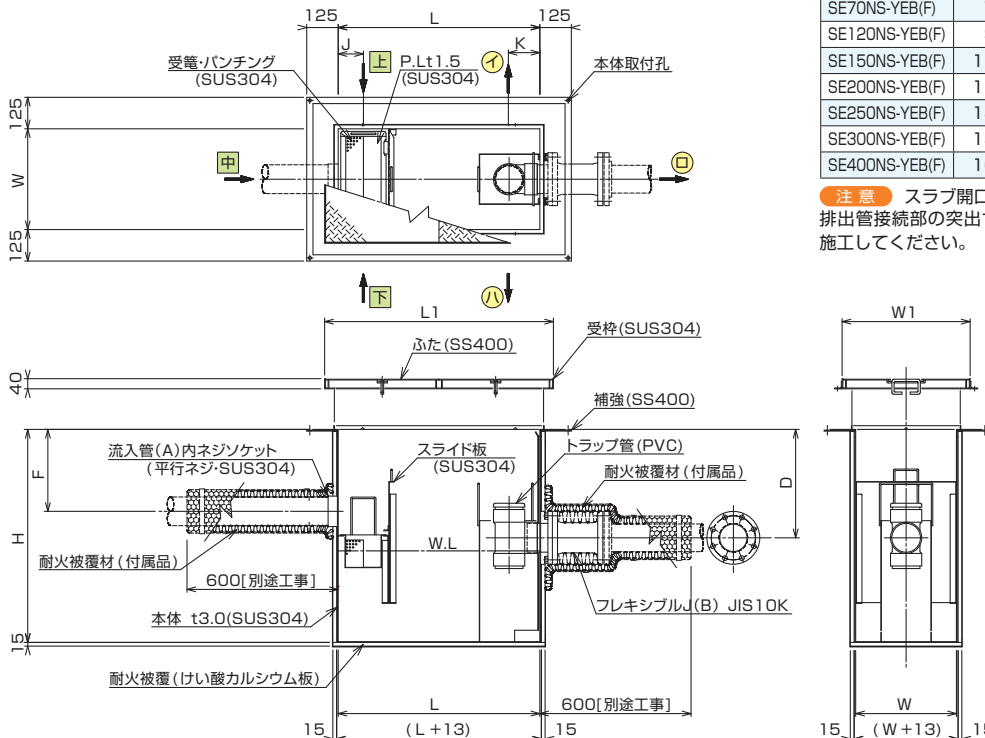
構造図
