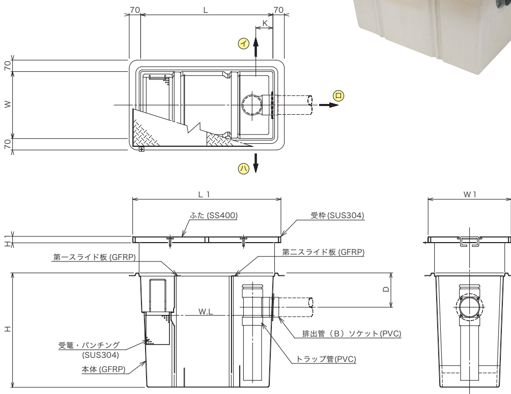
構造図
