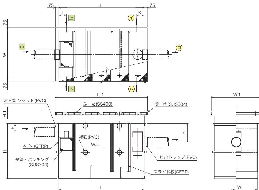
構造図
