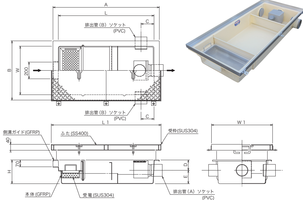
構造図
