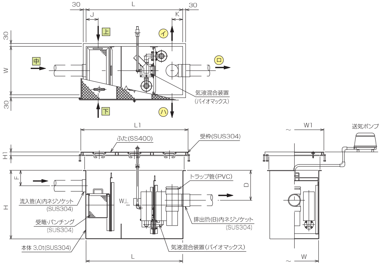
構造図
