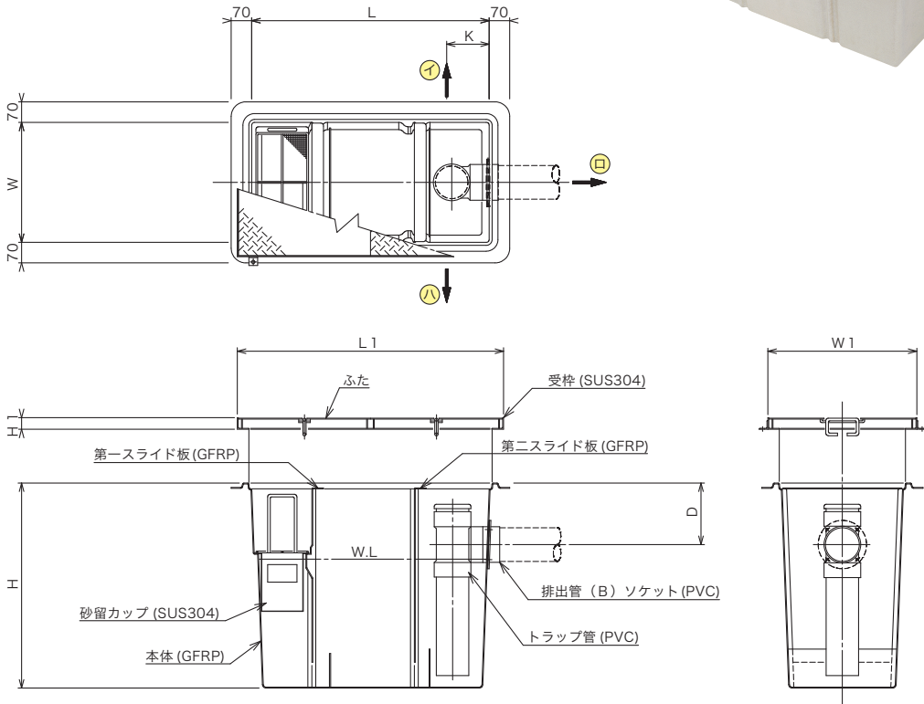
構造図
