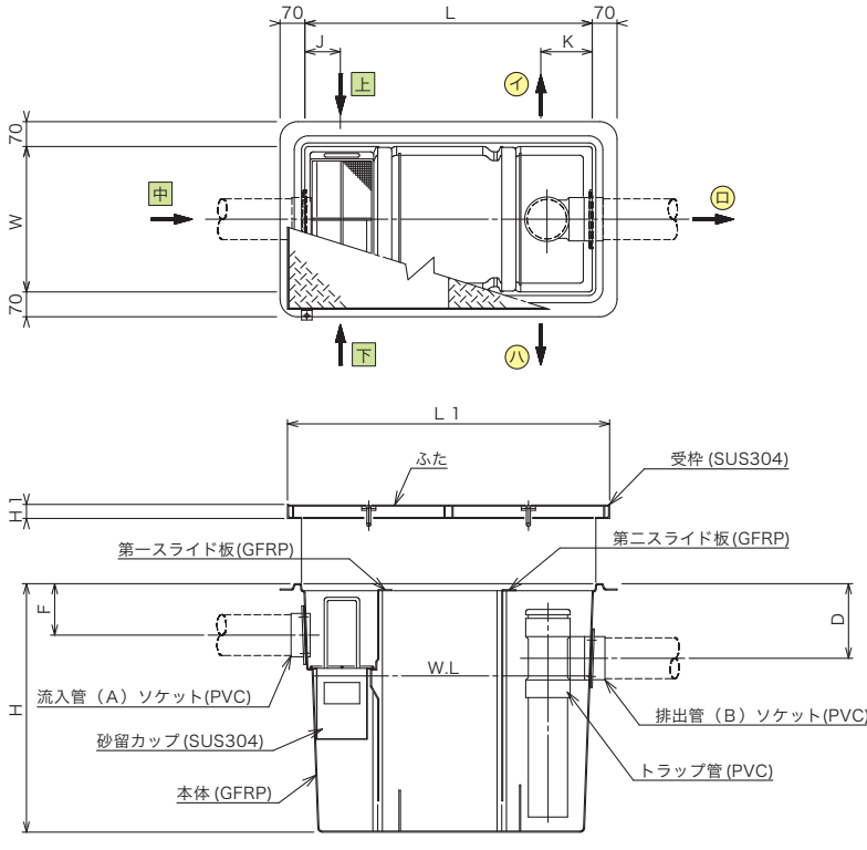
構造図
