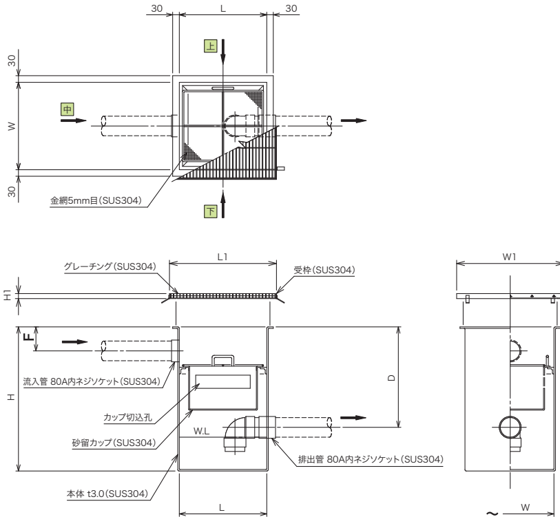
構造図
