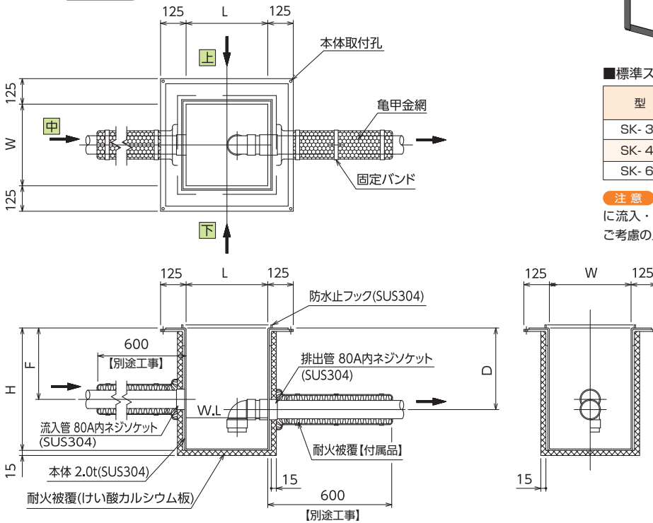
構造図
