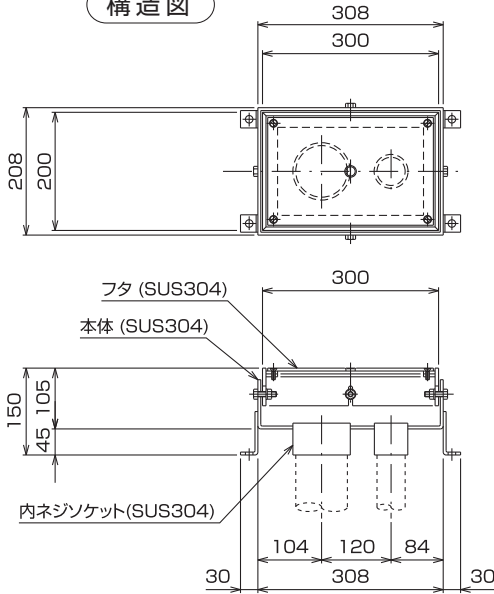
構造図
