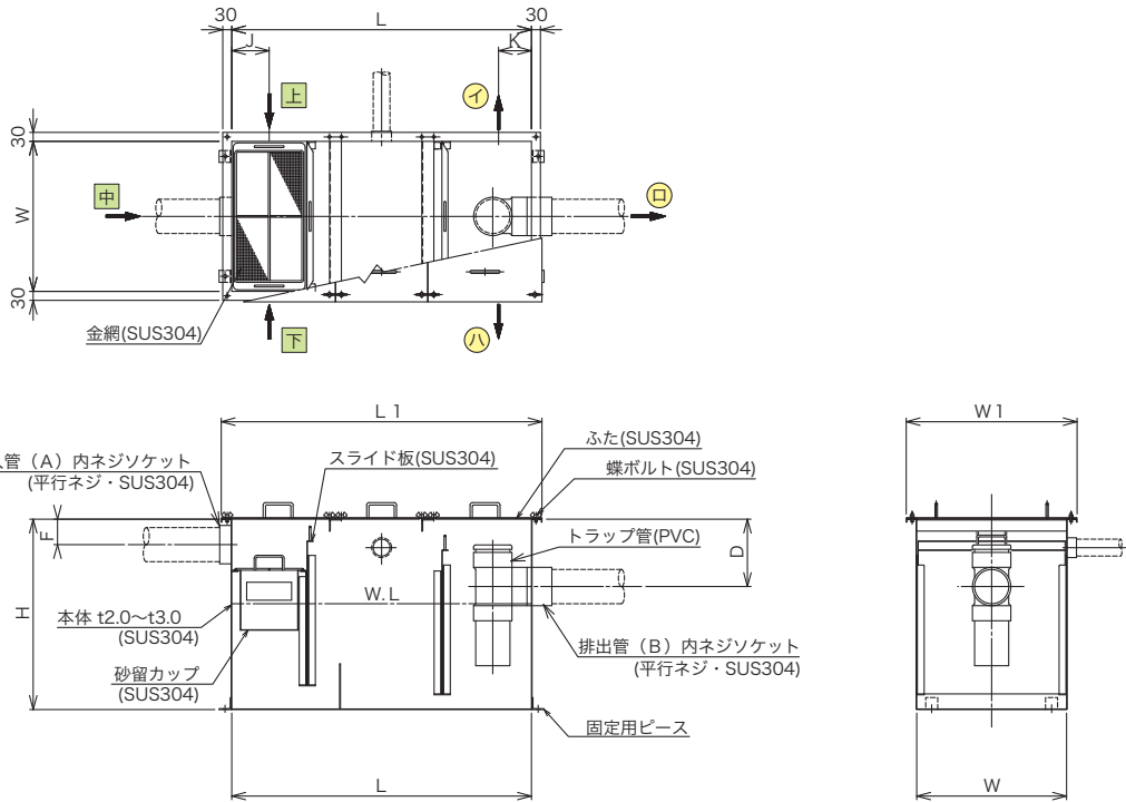
構造図
